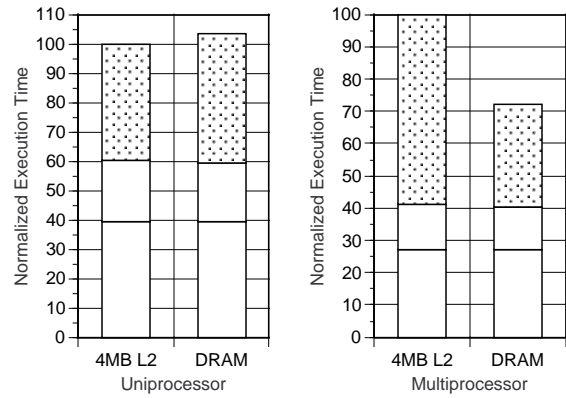
(d) eqntott:
